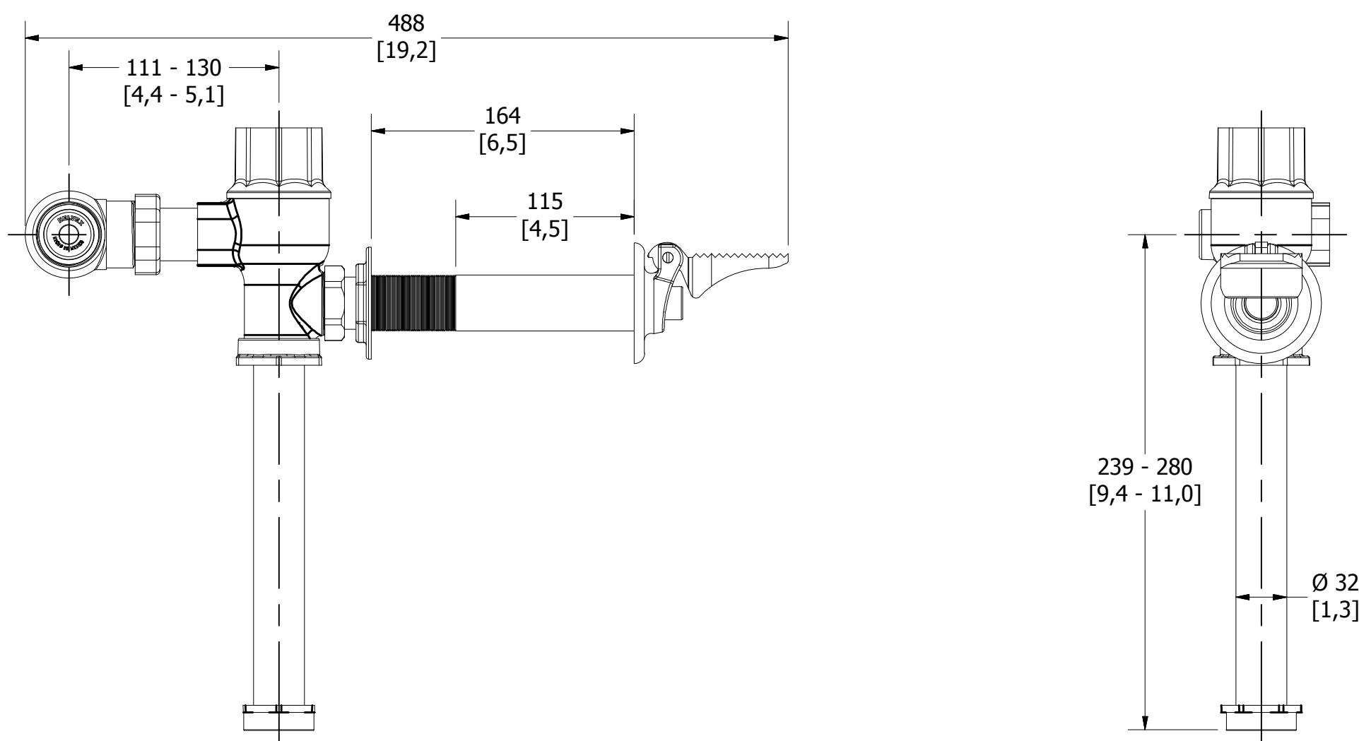
Medidas Referenciales / Estimated Dimensions, Acot.mm.[pulg] / Dim.mm.[in]
