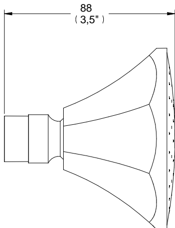
Medidas Referenciales / Estimated Dimensions, Acot.mm (pulgadas) / Dim.mm (inches)
