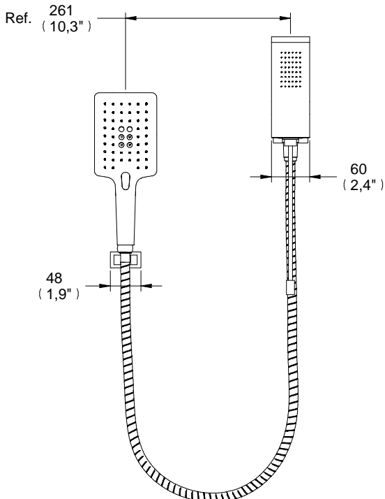
Medidas Referenciales / Estimated Dimensions, Acot.mm.(pulg) / Dim.mm.(in)
